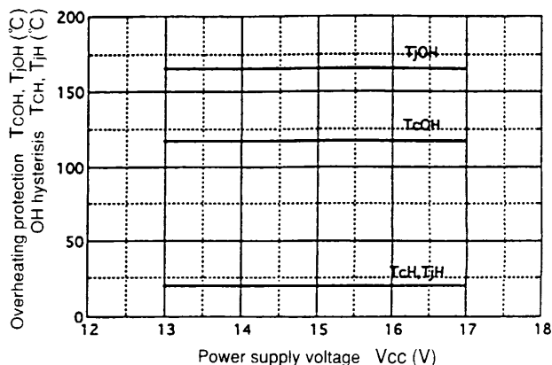
過熱保護動作温度ー電源電圧特性 Overheating characteristics T_{COH} , T_{jOH} , T_{CH} , T_{jH} vs. V_{CC}
