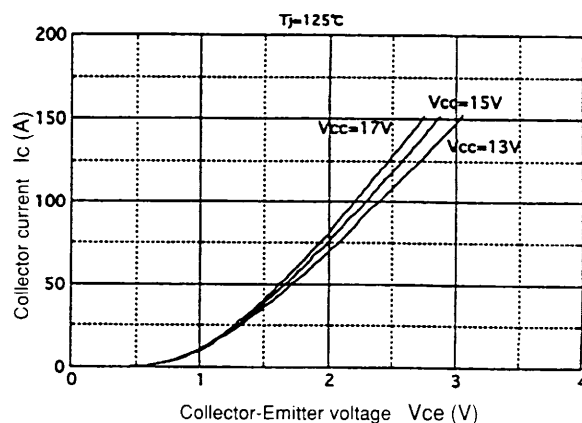
コレクタ電流ーコレクタ・エミッタ間電圧特性 Collector current vs. Collector-Emitter voltage
