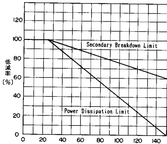
ASO 低減特性 ASO Derating
